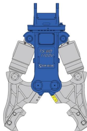
【新製品】TS-WD1100VR(ツース交換式)
